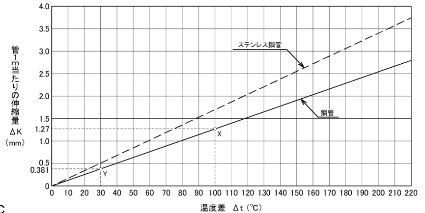
図 管の1m当りの伸縮量
