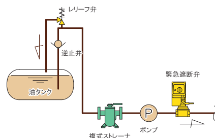
図2.給油配管例
