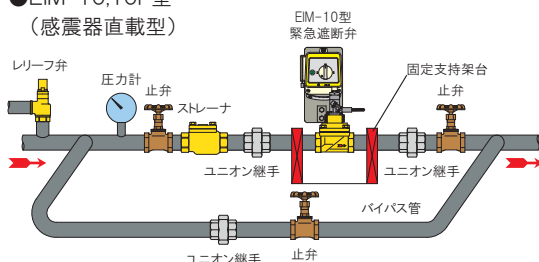
図1.配管例略図
