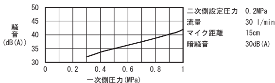
一次側圧力変化時の騒音特性
