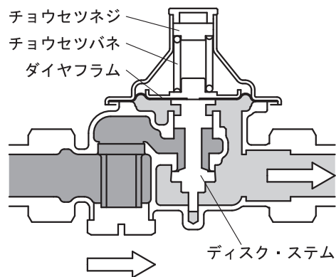
『弁閉』
