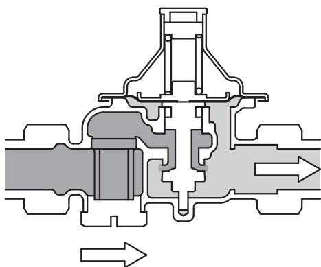
『弁開』
