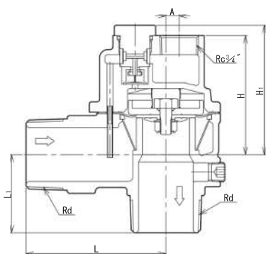
LP-8AN Type
