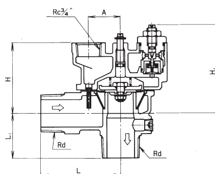
LP-8AHN Type
