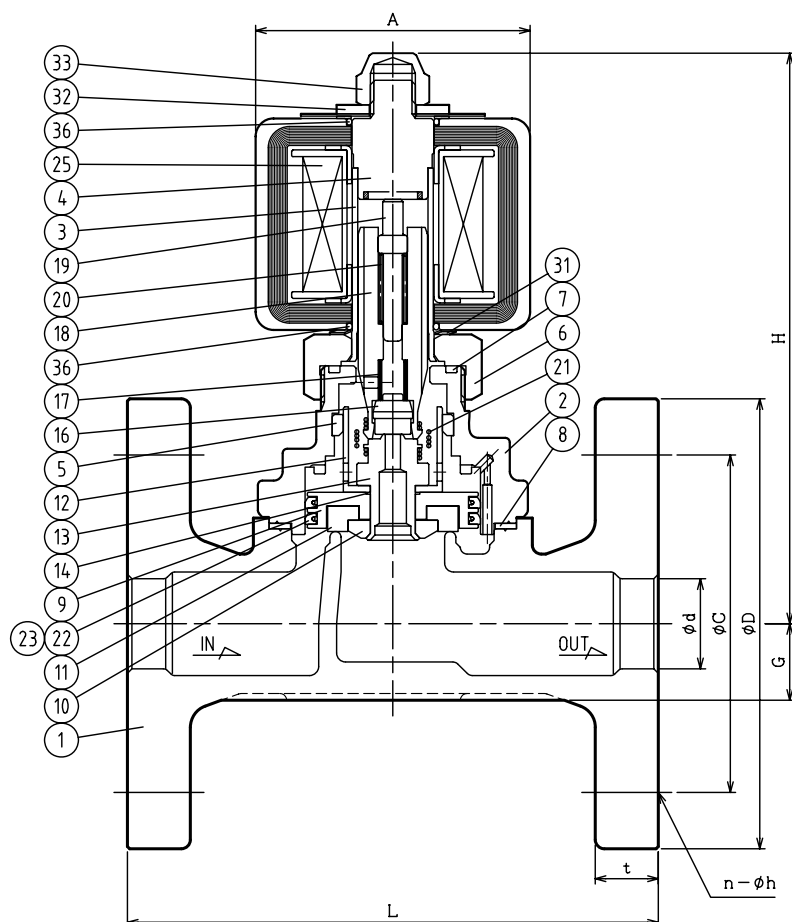
TB-03C型の場合
