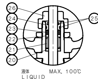
矢視 (A) 部 パッキングランド部構造 CONSTRUCTION OF PACKING GLAND (A) PORTION ABOVE
