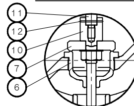
SIZE 40~50mm DISC (METAL TOUCH DISC)
