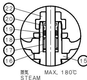
矢視 (A) 部 パッキングランド部構造 CONSTRUCTION OF PACKING GLAND (A PORTION ABOVE)
