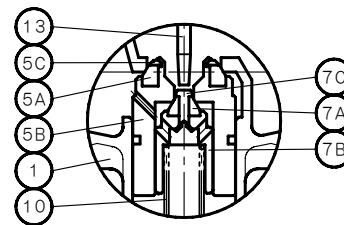
テフロンディスク入り構造 PTFE SEAL IN PLUG
