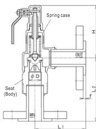
SL-39F Type
