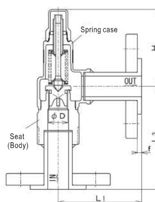
SL-40F Type
