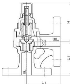
SL-44E Type
