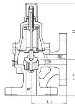
SL-24E Type
