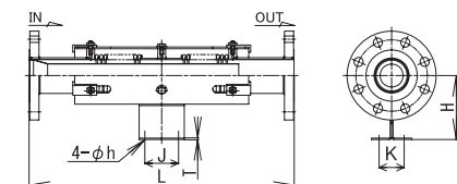
JB-32型
