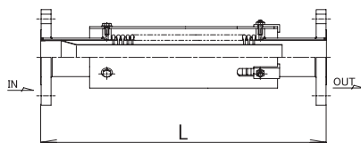
JB-32型
