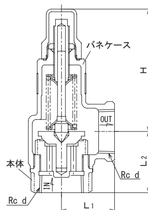
SL-40E,40EN型
