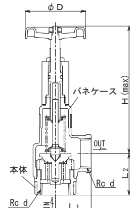
SL-40EA型
