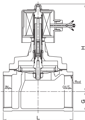
WS-12,12N型
