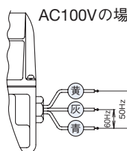
AC100Vの場合
