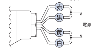
AC100/110Vの場合
