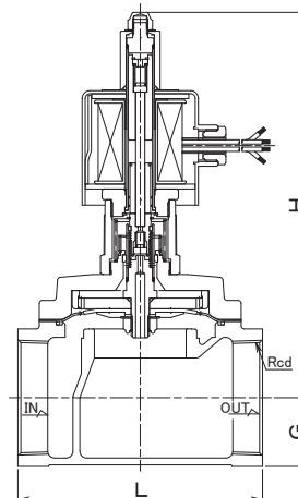
WS-12C,12CN型
