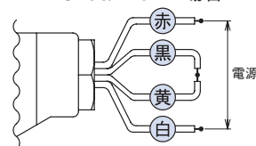
AC200/220Vの場合
