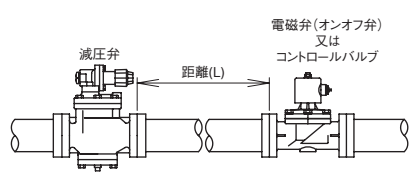
図3. 減圧弁と制御弁との距離
