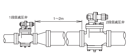
図4. 二段減圧弁での弁間隔
