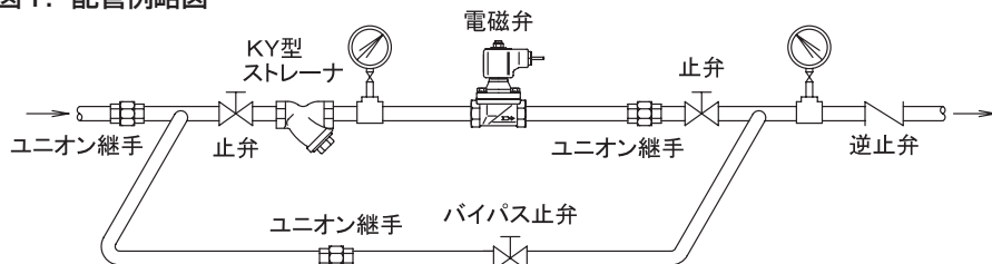
図1. 配管例略図
