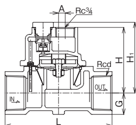
呼び径25～50 (LP-8N型)
