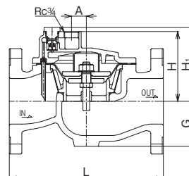
呼び径65～100 (LP-8N, 9N型)
