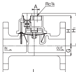
呼び径40・50 (LP-9N型)
