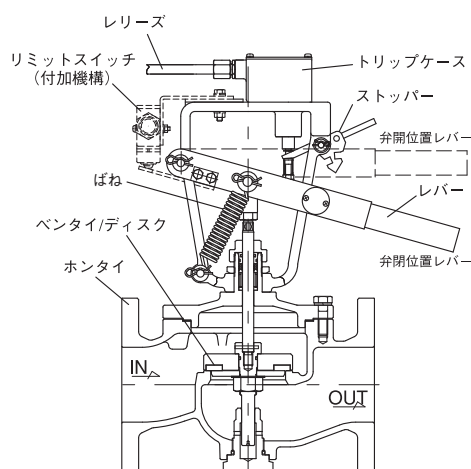
図1. 本体部
