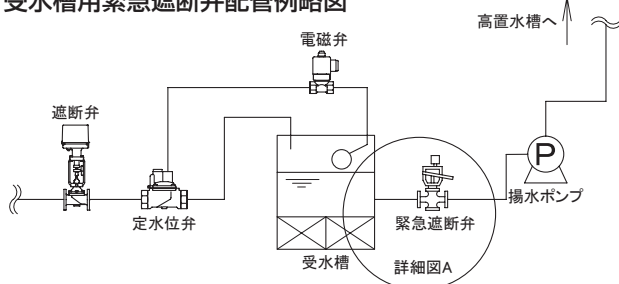
図3. 受水槽用緊急遮断弁配管例略図
