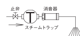
図6. 大気開放配管例略図
