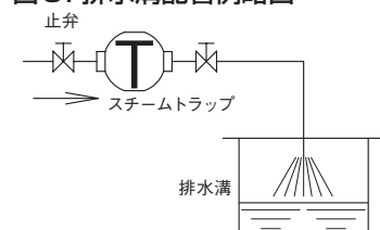
図5. 排水溝配管例略図
