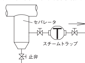
図2. 配管途中取付例略図
