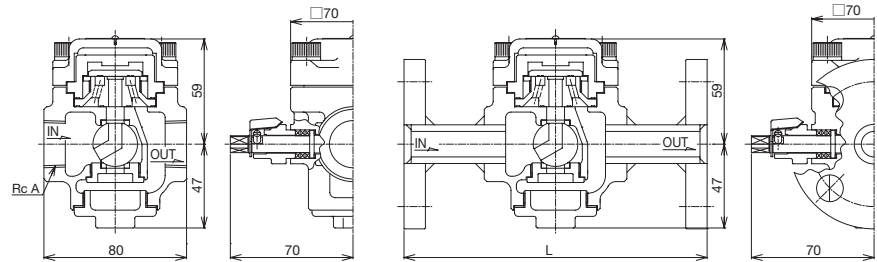
ADB-21型
