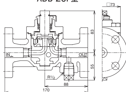
ADB-20F型
