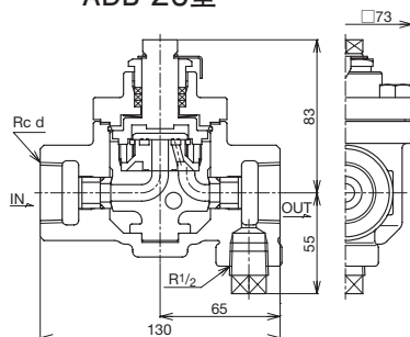
ADB-20型
