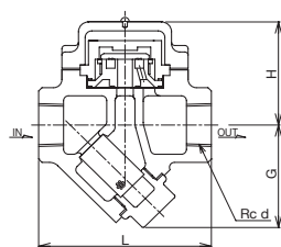
AD-19型
