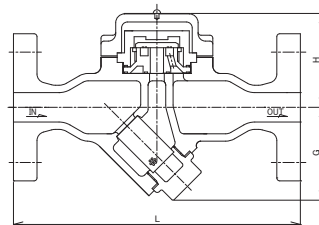
AD-19F型
