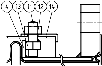
矢視 (A) 部 ( (A) PORTION ABOVE )
