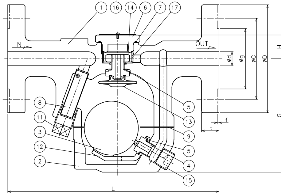
DEMENSIONS (mm) FLANGE CODE: JIS 10K, 16K, 20K共用フランジ
