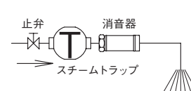
図6. 大気開放配管例略図
