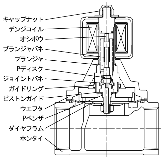
WS-22V型（呼び径32～50）構造図
