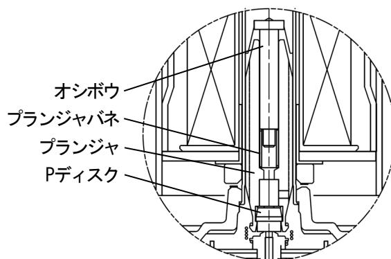
DC用の場合のプランジャ部分 (呼び径10～50)
