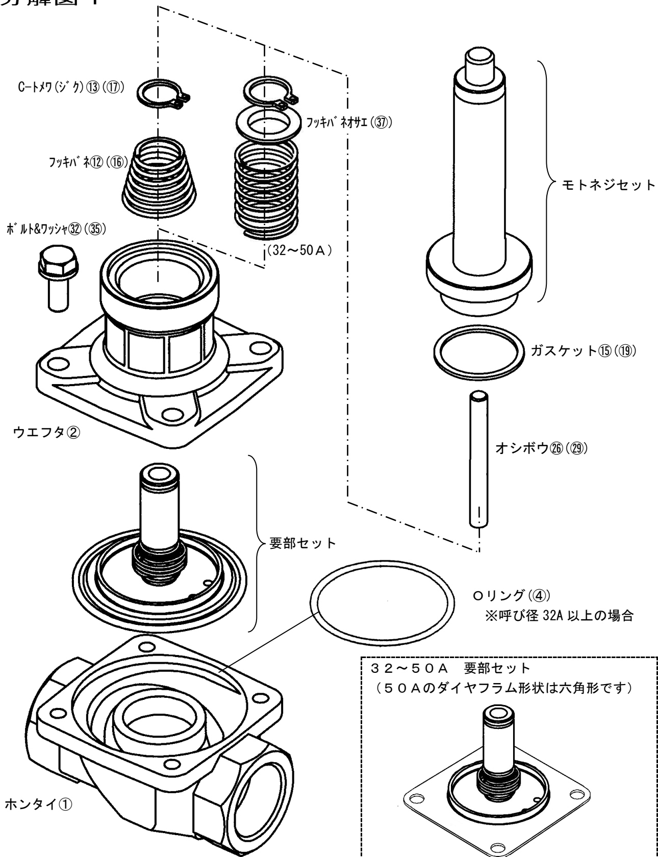
分解図 1
