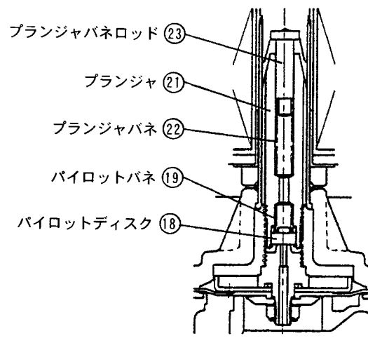
DC用の場合のプランジャ部分
