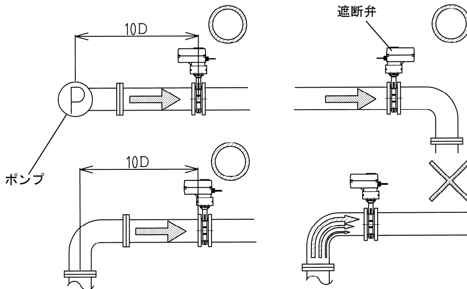
図 2-3 : ポンプ出口側の取付・曲がり管への取付
