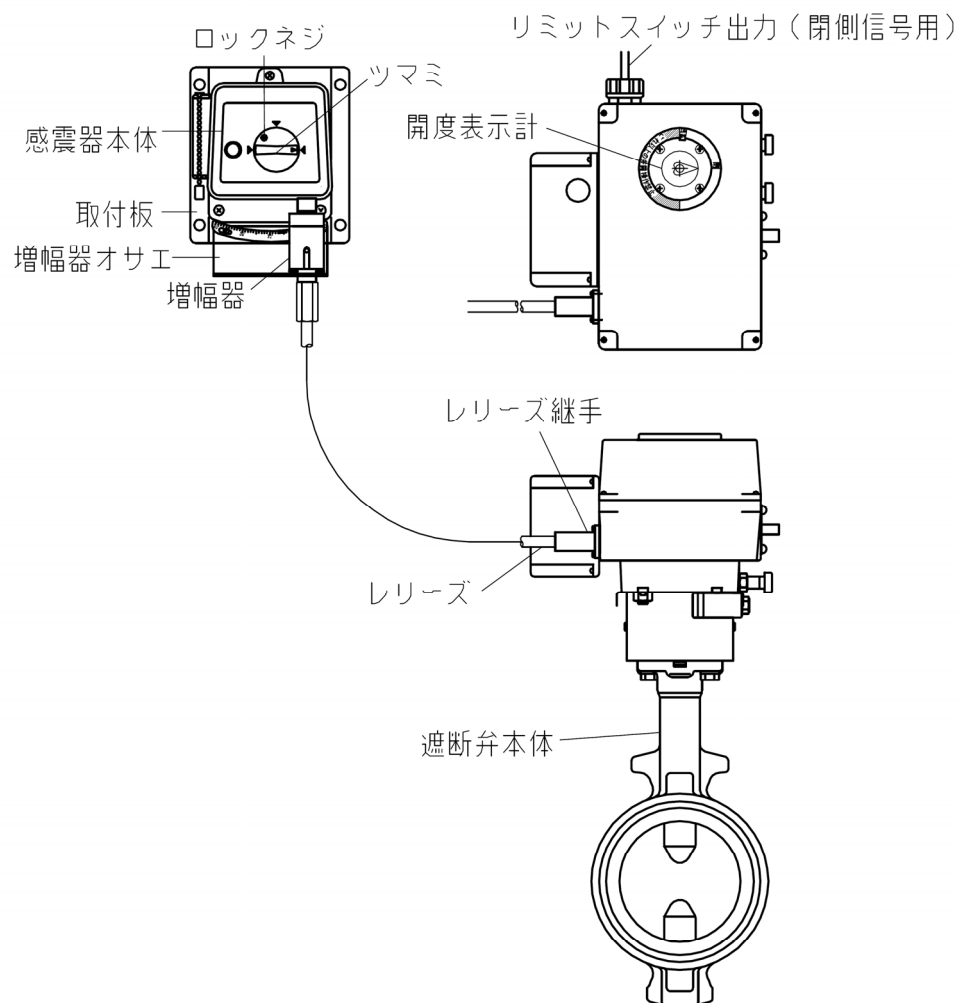
図 1 - 1 : 機械式遮断弁システム図
