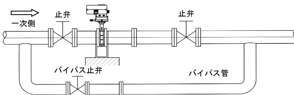
図 2-2 : 側路 (バイパス) を組む場合
