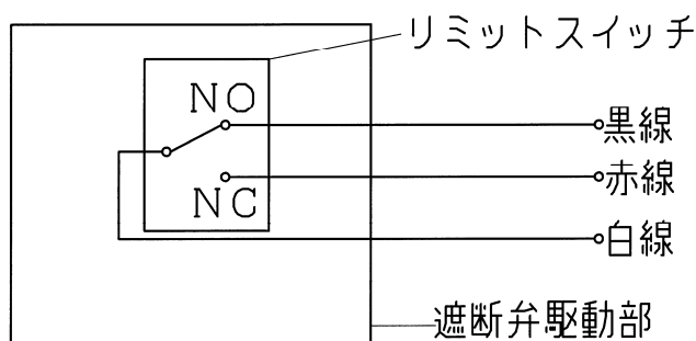
図 2-13 : リミットスイッチ
