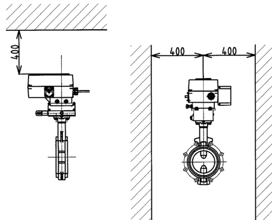
図 2-4 メンテナンススペース
