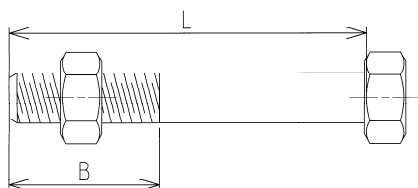
図 2-5 : 六角ボルト図
