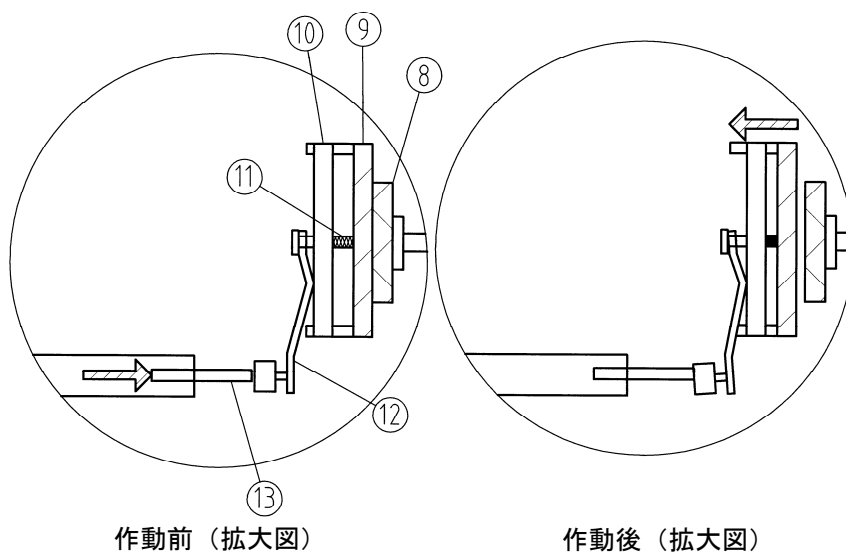
図 1－5：作動図
