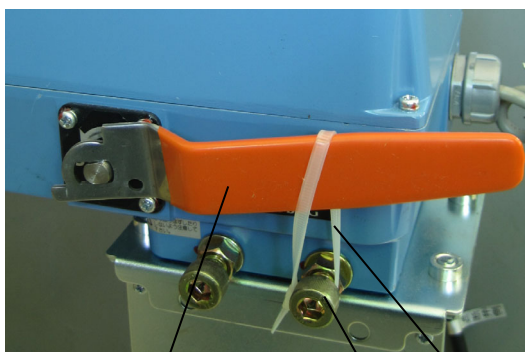
復帰ハンドル ボルト 結束バンド 図 4 - 2 : 応急処置方法 (結束バンド使用方法)
