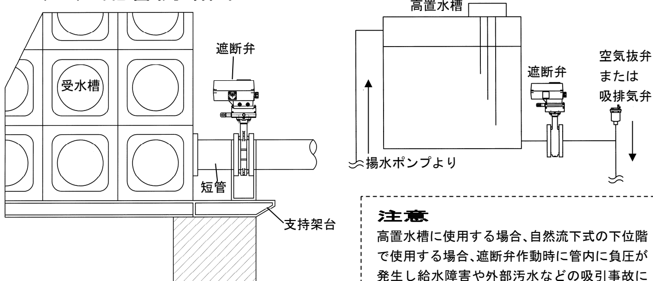
図 2-1 : 受水槽設置配管例と高置水槽設置配管例
