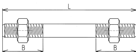
図 2-6 : 両ねじボルト図
