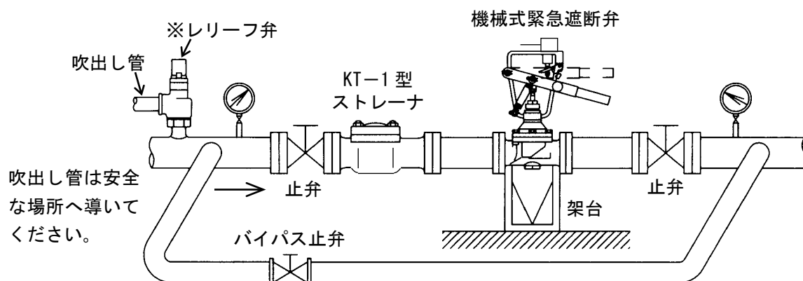
図2-2：給油配管例
