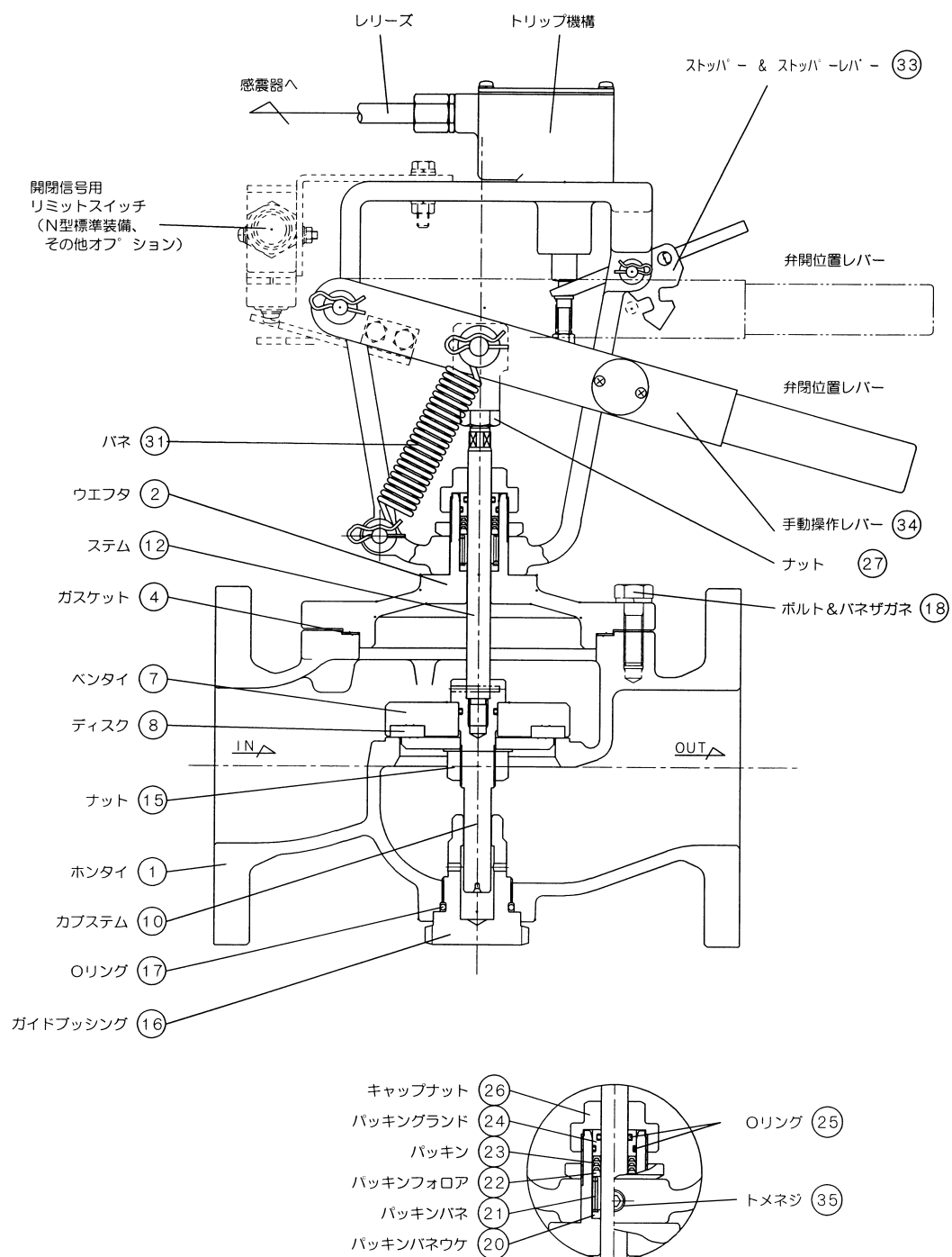
図1-4：構造図
