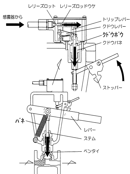
図１－６：作動図＜弁閉状態＞
