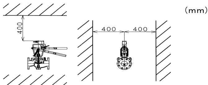
図2-5：メンテナンススペース
