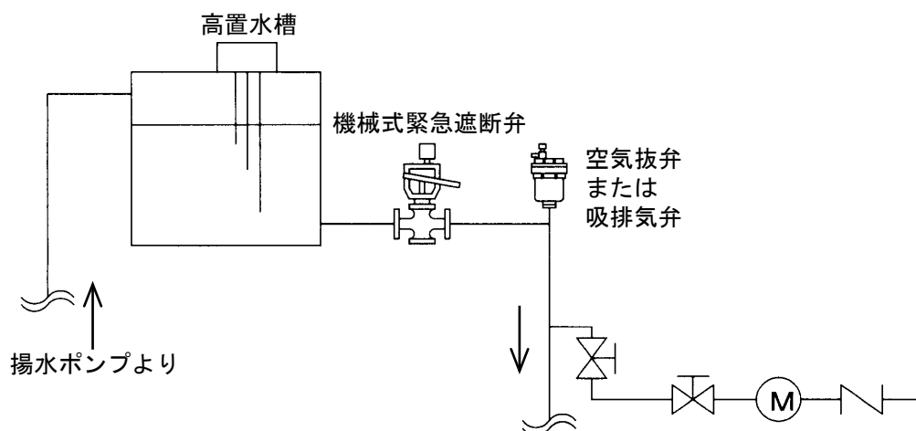
図 2－4：高置水槽設置配管例
