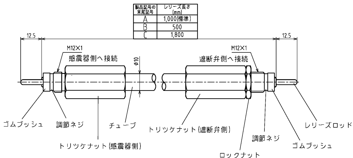
図 1 - 3 : レリース構造図 (ロックナットを組込んである方を遮断弁に接続。)
