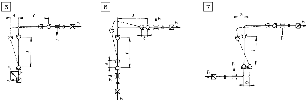
ボールジョイント間の距離 \ell (安全率1.5)
