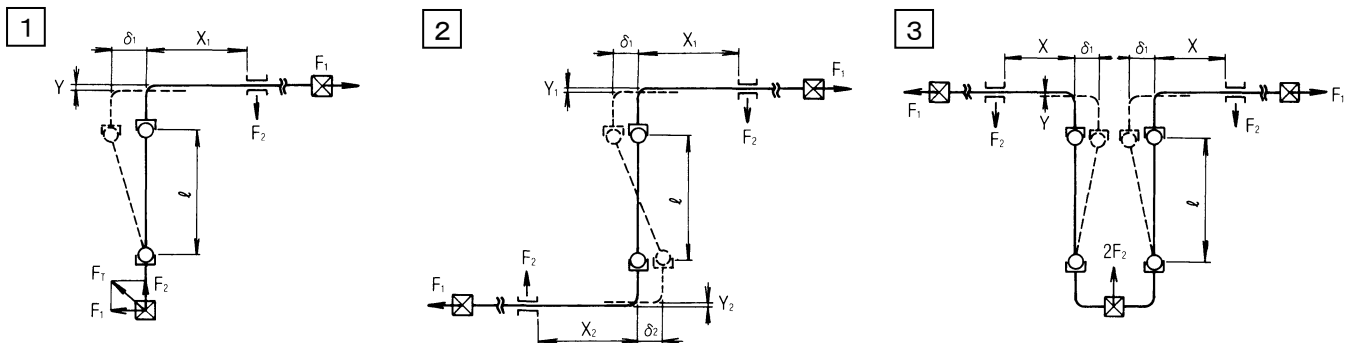
ボールジョイント間の距離 \ell (安全率1.5)
