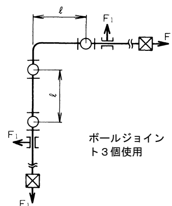
図7 直角配管での伸縮
