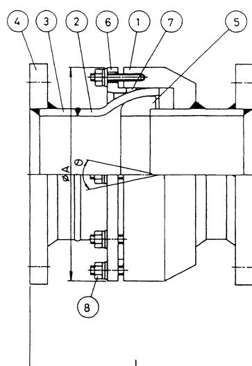
J U - 3 F 型, 4 F 型
