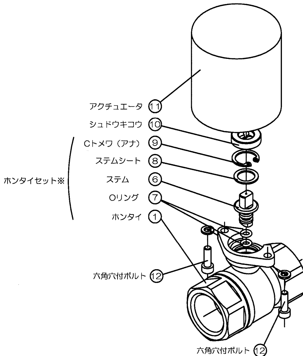
分解図 １
