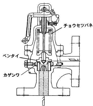
図 1 弁閉
