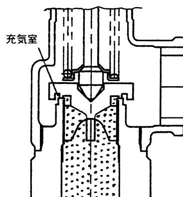
図 2 吹始め
