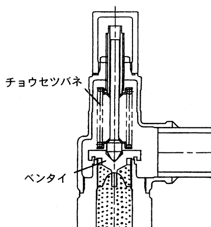
図 1 弁閉
