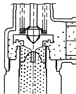
図 3 全開 (→弁閉)
