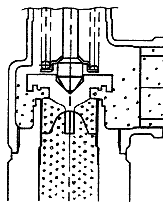
図 3 全開 (→弁閉)
