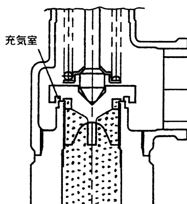
図 2 吹始め
