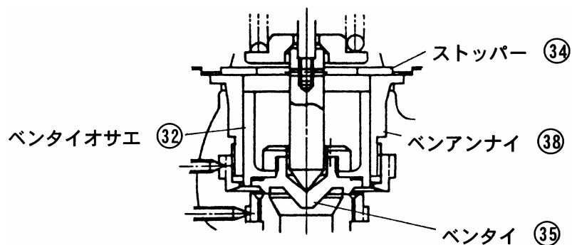
SF-19L型
