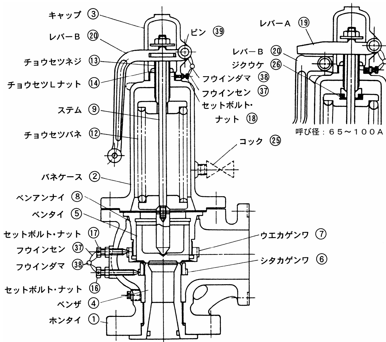
SF-19型
