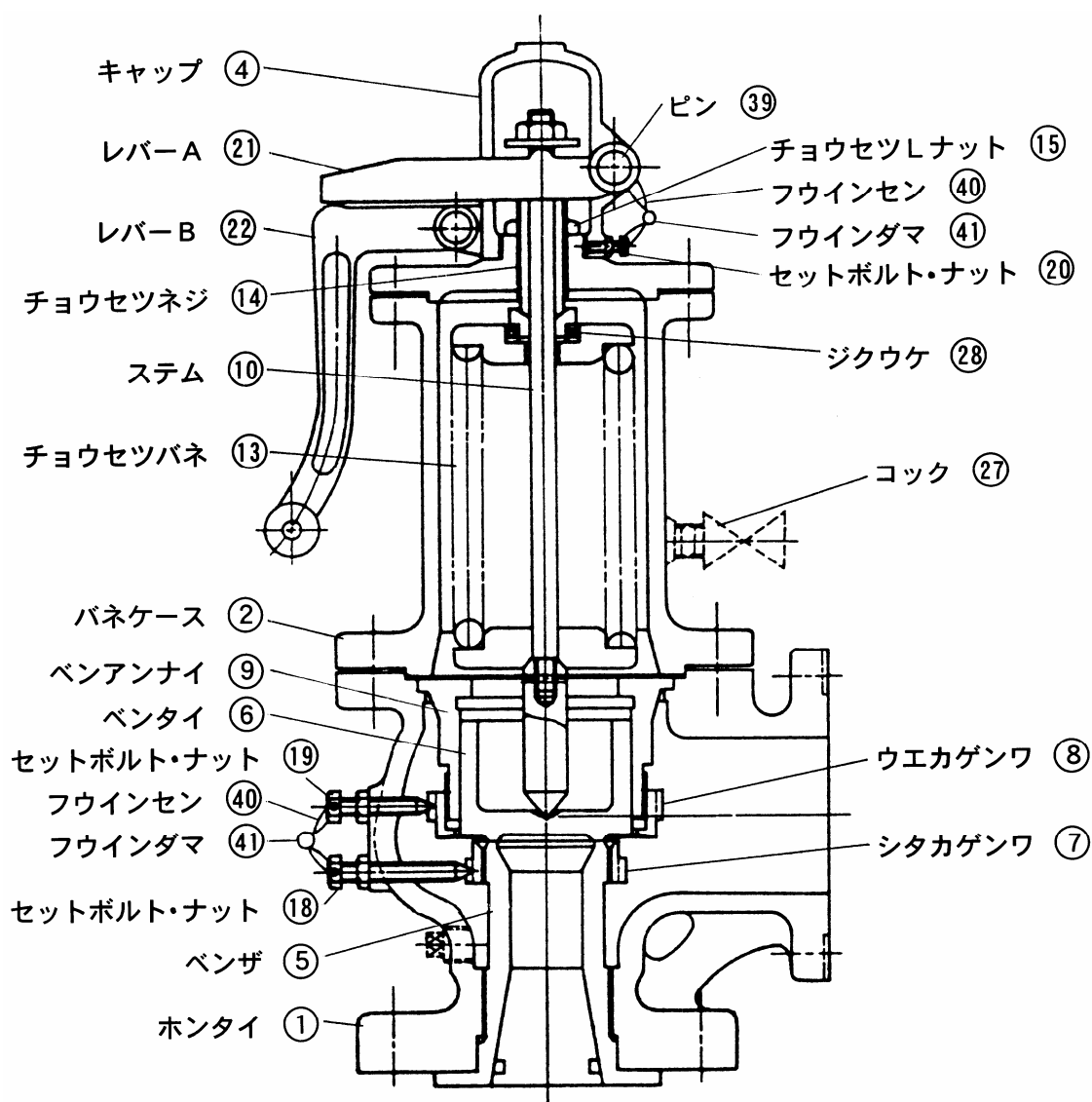
SF-19型
