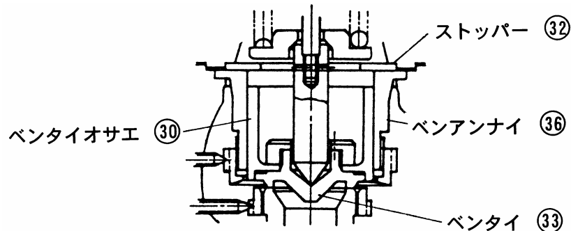
SF-19L型
