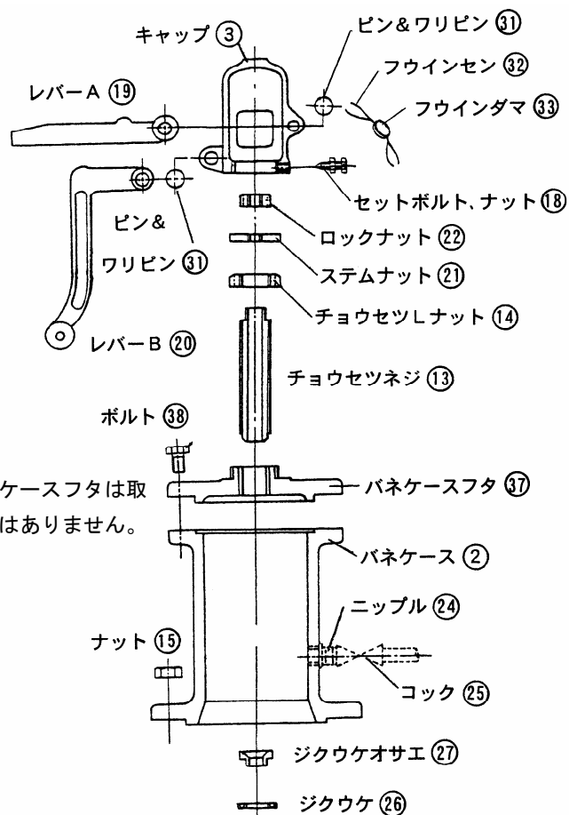
SF-15型 (呼び径: 150)
