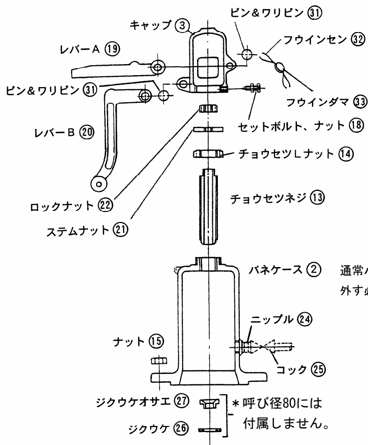
SF-15型 (呼び径: 80~125)
