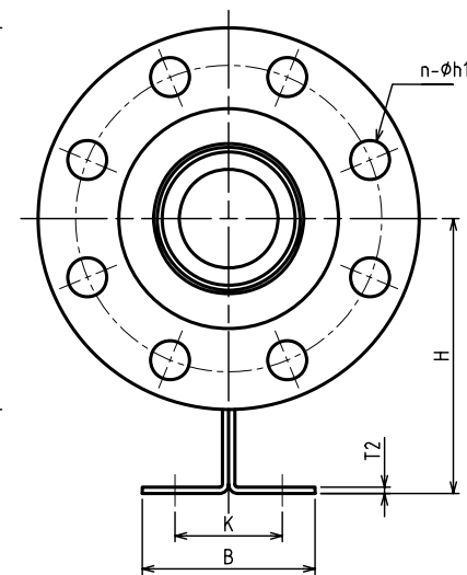
矢視(B)部 (B) PORTION ABOVE)
