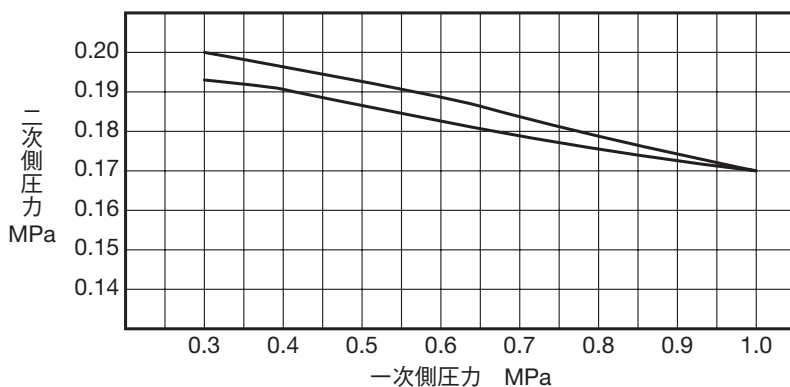
一次側圧力0.3MPaの時、二次側圧力を0.2MPaに設定後、一次側圧力を0.3~1.0~0.3MPaに変化させた時の二次側圧力の変動を示します。
