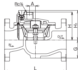
呼び径65～100 (LP-8N, 9N型)
