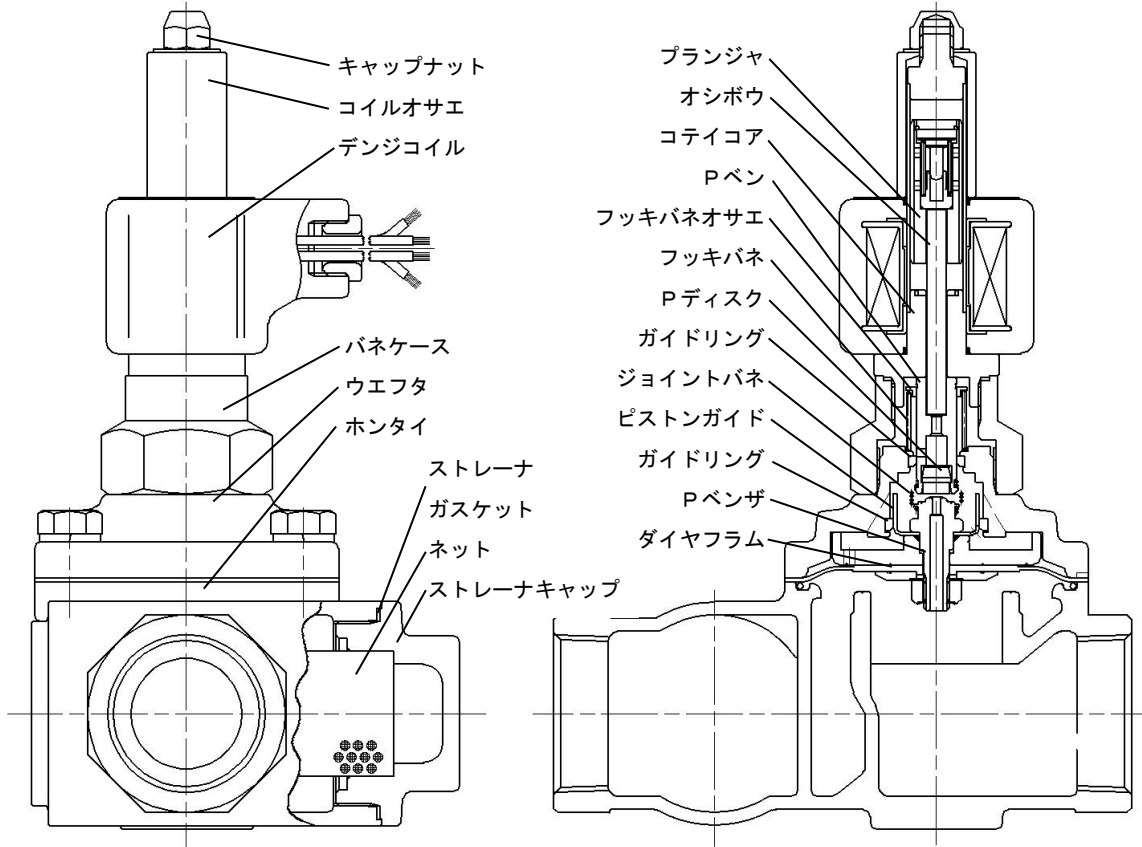
WS-43C (呼び径32~50) 構造図
