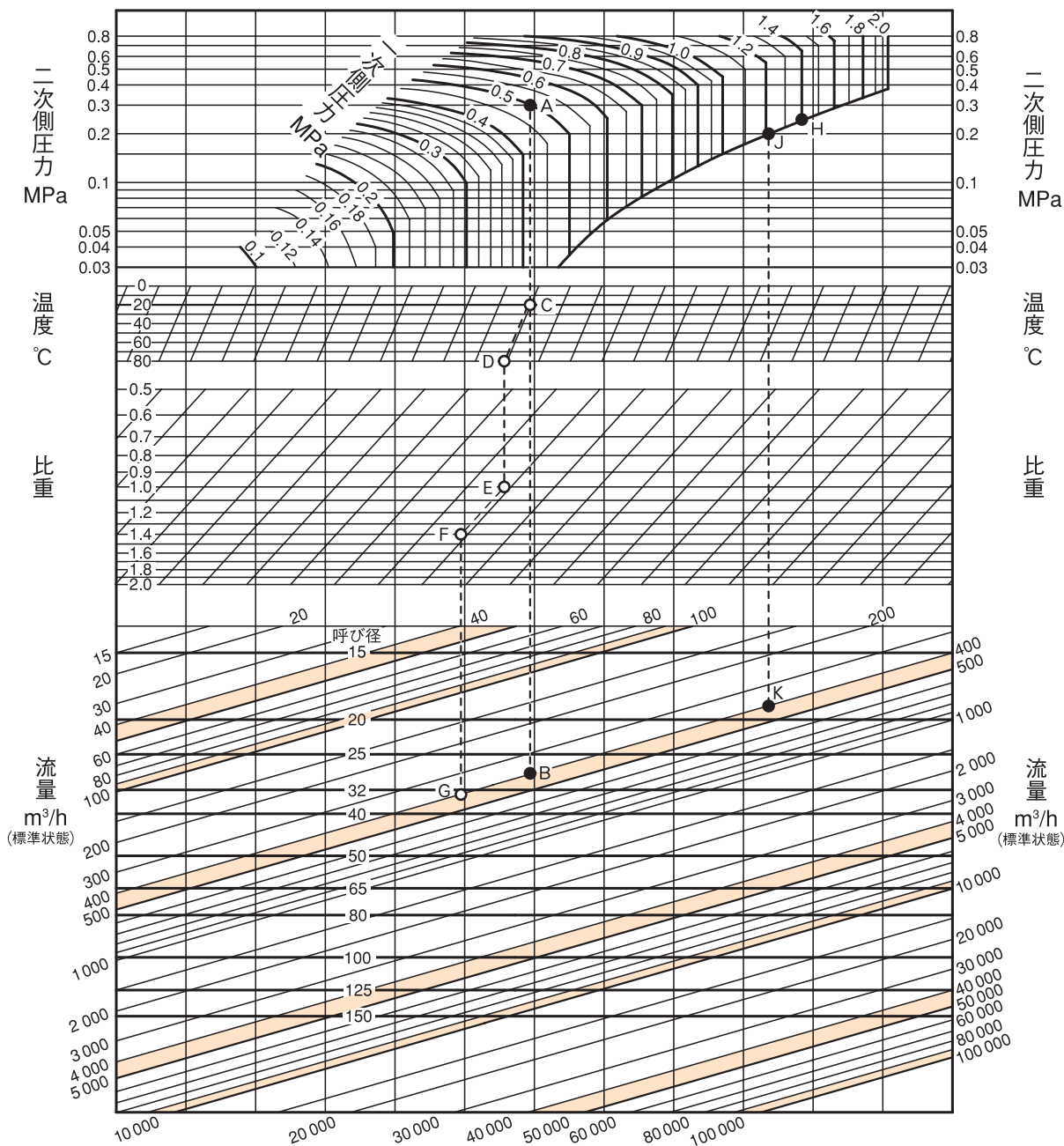
呼び径選定図表(気体用)
