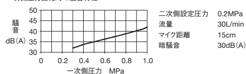
一次側圧力変化時の騒音特性
