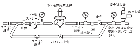
図3. 端接続がねじ込形的場合
