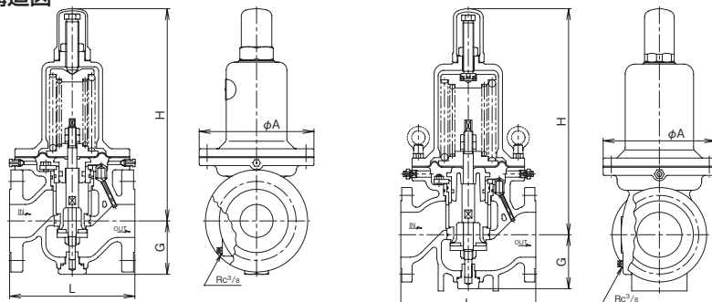
呼び径15～80
