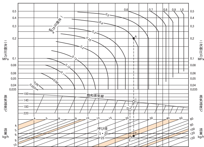
RD-3H,3HF型呼び径選定図表<蒸気用>
