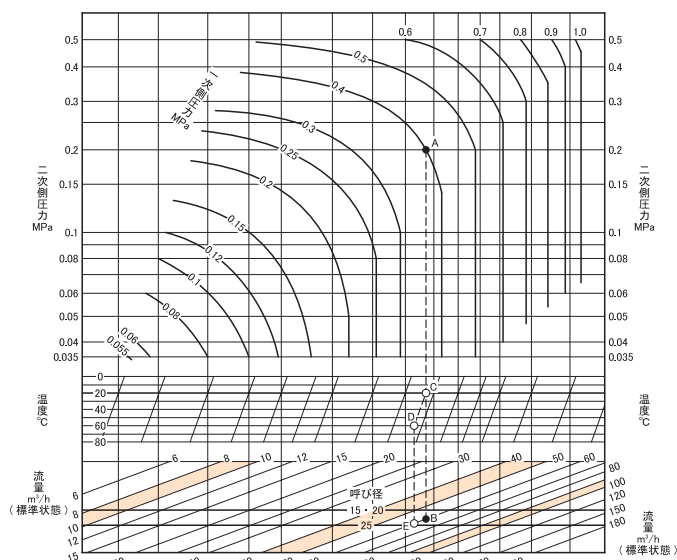
RD-3HA,3HAF型呼び径選定図表<空気用>
