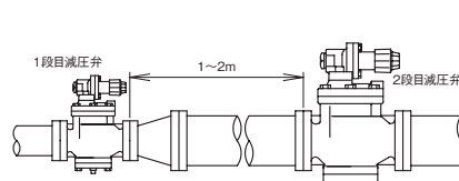
図4. 二段減圧弁での弁間隔
