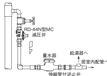
オス・メスユニオン継手の場合
