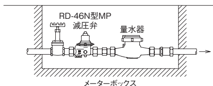
量水器一次側 取付例
