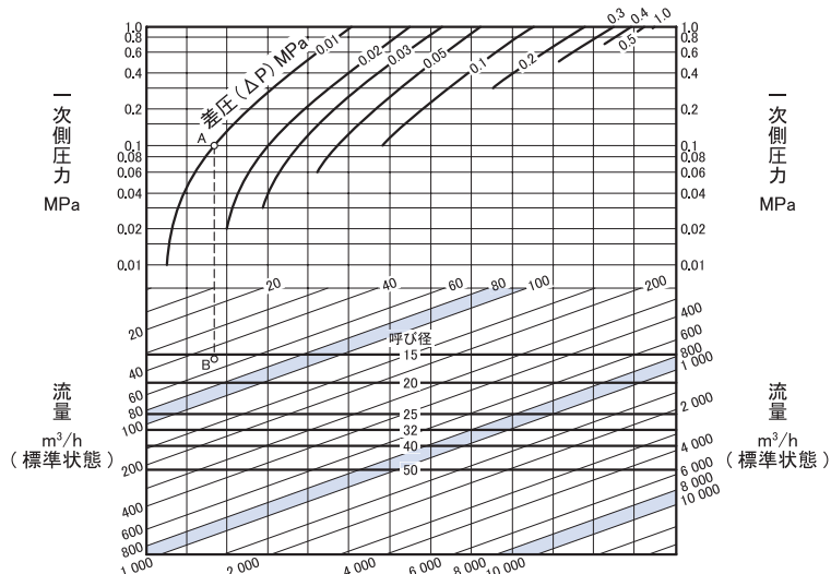
呼び径選定図表<空気用>
