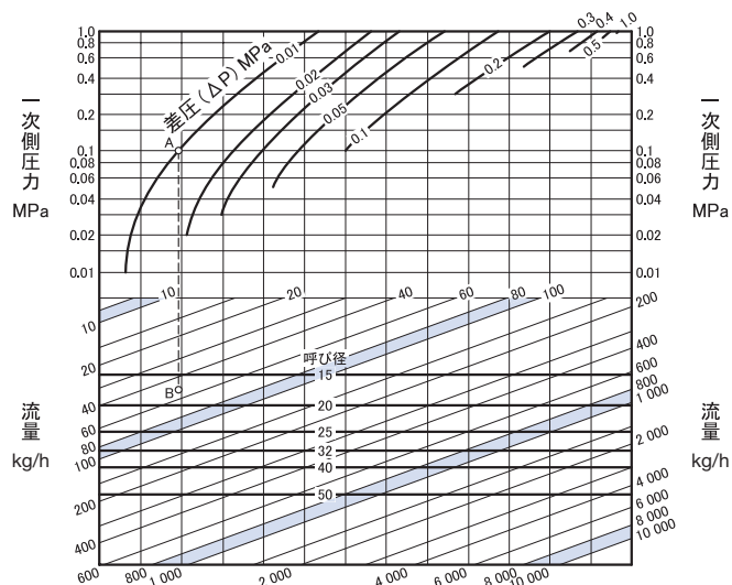
呼び径選定図表<水用>
