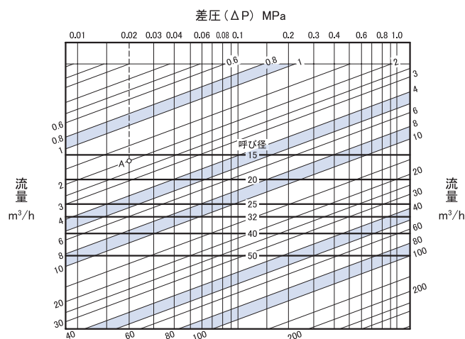
呼び径選定図表<空気用>
