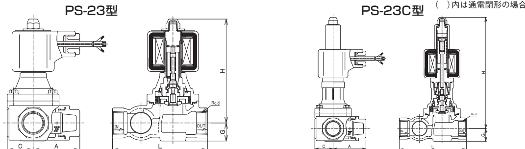
PS-23C型 (呼び径 32~50)
